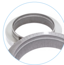
Spannungswellengetriebe Material: 100Cr6 Tiefe: 7 mm Prozesszeit: 23 min. Ra: 0,4 µm
